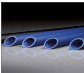
Materiale: Fusiolen PP-R / PP-RCT Colore: blu Applicazione: riscaldamento, condizionamento refrigerazione NON UTILIZZABILE PER IL TRASPORTO DI ACQUA POTABILE
